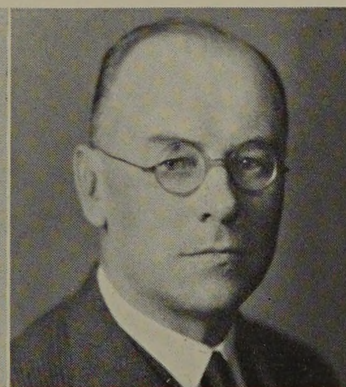
H. Tropsch
