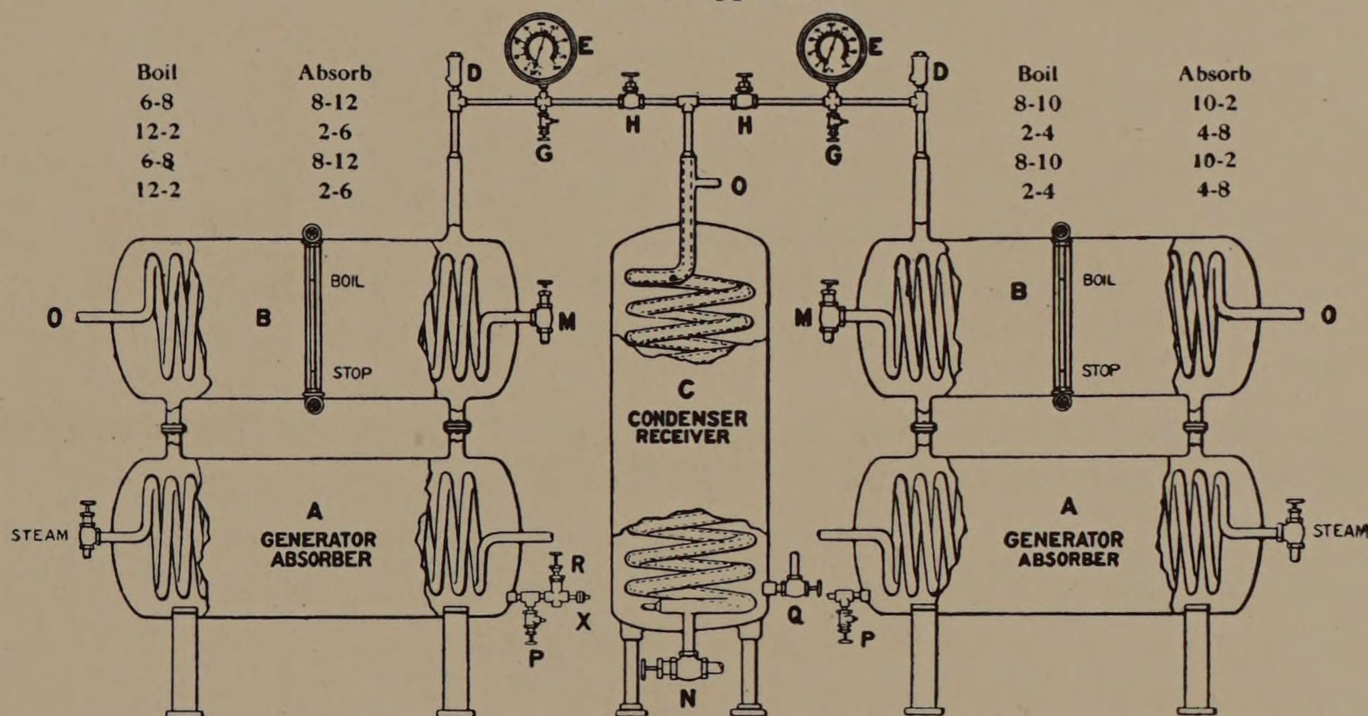
Double Apparatus
